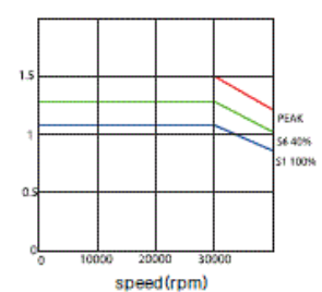
Torque(Nm)
