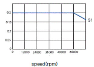
Torque (Nm)
