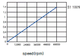
Power(Kw)
